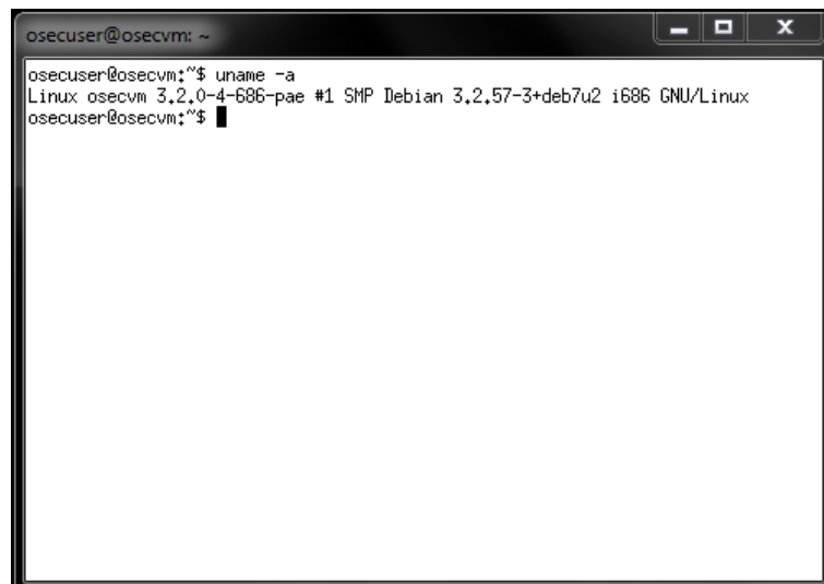
Figure 10: XTerm Anwendungsfenster
